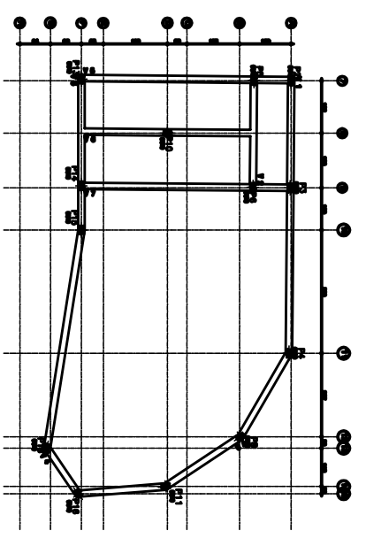
PLANTA FORMA - BALCONIE 2 Esc: 1:50
